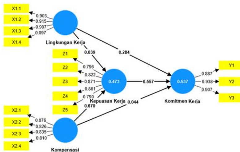
Gambar 1 Algoritem
