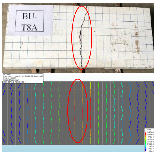
Gambar 16. Pola retak hasil eksperimen vs diana fea T-100mm (Sumber : Pengolahan data, 2022).
