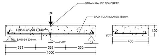
Gambar 4. Skema pembebanan benda uji (T-120 mm) (Sumber : Penulis, 2022)
