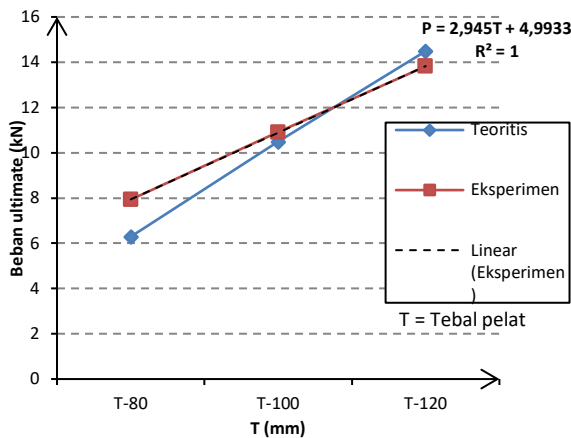
Gambar 10. Diagram perbandingan beban retak awal hasil teoritis dan eksperimen (Sumber : Pengolahan data, 2022).
