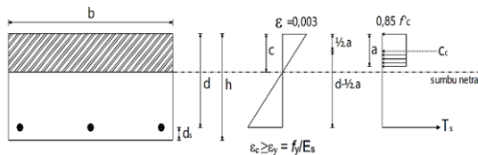
Gambar 1. Diagram regangan dan gaya pada pelat penampang solid. (Sumber : Dipohusodo, I., 1999)
