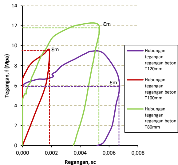
Gambar 9. Gabungan grafik hubungan tegangan dan regangan beton pelat (Eksperimen)
