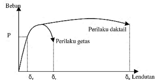
Gambar 2. Grafik beban-lendutan pelat beton bertulang. (Sumber : Ujjianto, M. 2006).
