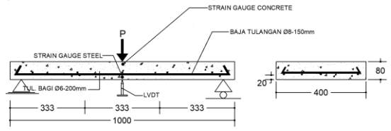
Gambar 6. Skema pembebanan benda uji (T-80 mm) (Sumber : Penulis, 2022)
