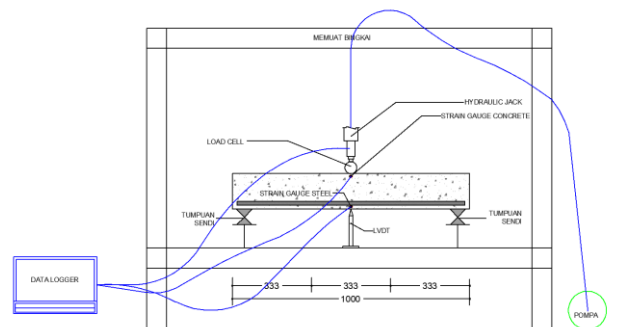
Gambar 7. Set up uji lentur Pelat. (Sumber : Penulis, 2022)
