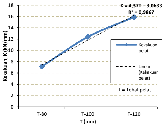
Gambar 12. Diagram kekakuan pelat eksperimen (Sumber : Pengolahan data, 2022).
