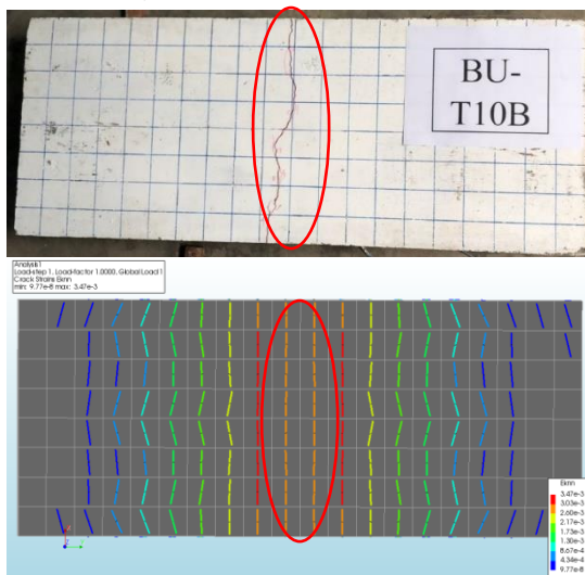
Gambar 15. Pola retak hasil eksperimen vs diana fea T-100mm (Sumber : Pengolahan data, 2022).
