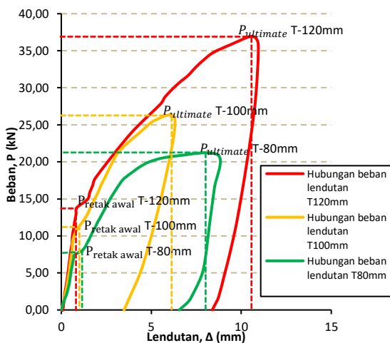
Gambar 8. Gabungan grafik hubungan beban dan lendutan pelat (Eksperimen) (Sumber : Pengolahan data, 2022).
