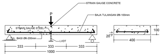
Gambar 5. Skema pembebanan benda uji (T-100 mm) (Sumber : Penulis, 2022)
