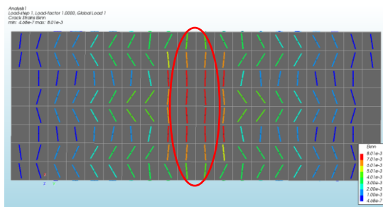
Gambar 14. Pola retak hasil eksperimen vs diana fea T-120mm (Sumber : Pengolahan data, 2022)
