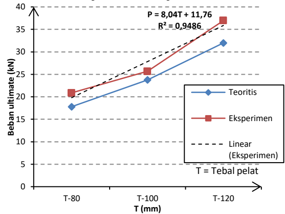
Gambar 11. Diagram perbandingan beban kapasitas hasil teoritis dan eksperimen (Sumber : Pengolahan data, 2022).
