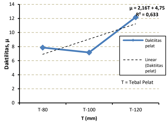
Gambar 13. Diagram daktilitas pelat eksperimen (Sumber : Pengolahan data, 2022).
