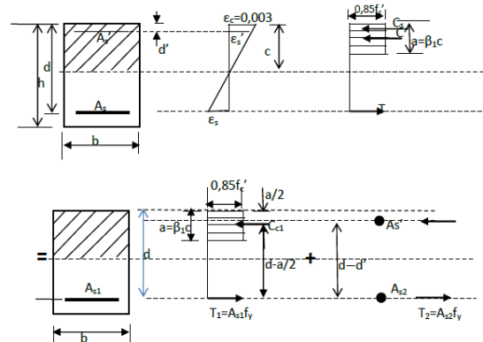
Gambar 2. Penampang balok tulangan rangkap dan analogi analisisnya.
