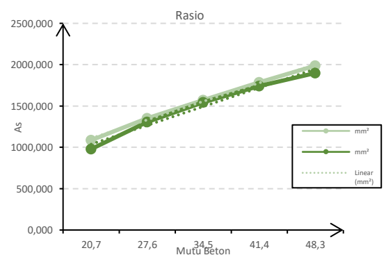
Gambar 10. Grafik nilai Rasio dengan Tulangan Rangkap dimensi 300 mm x 500 mm Sumber: Hasil Perhitungan,2022
