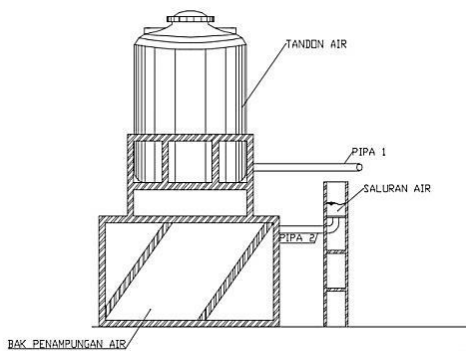
3. Potongan A-A
