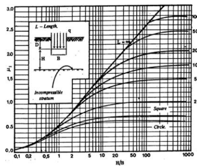
Gambar 11. Grafik Penentuan Nilai \mu_1 Sumber: Janbu, Bjerrum dan Kjaernsli (Hardiyatmo, 2010)
