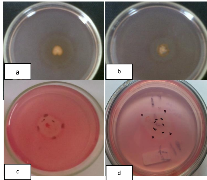
Gambar 4. Analisis kualitatif isolat bakteri pada media CMC 1% menggunakan metode Congo Red . Isolat yang memiliki Indeks zona bening terbesar a.) isolat 6.1 asal tanah kandang ayam, b) isolat 6.2 asal tanah kandang ayam, c) isolat 10.1 asal tanah sampah dan d) isolat 2.3 asal comberan.
